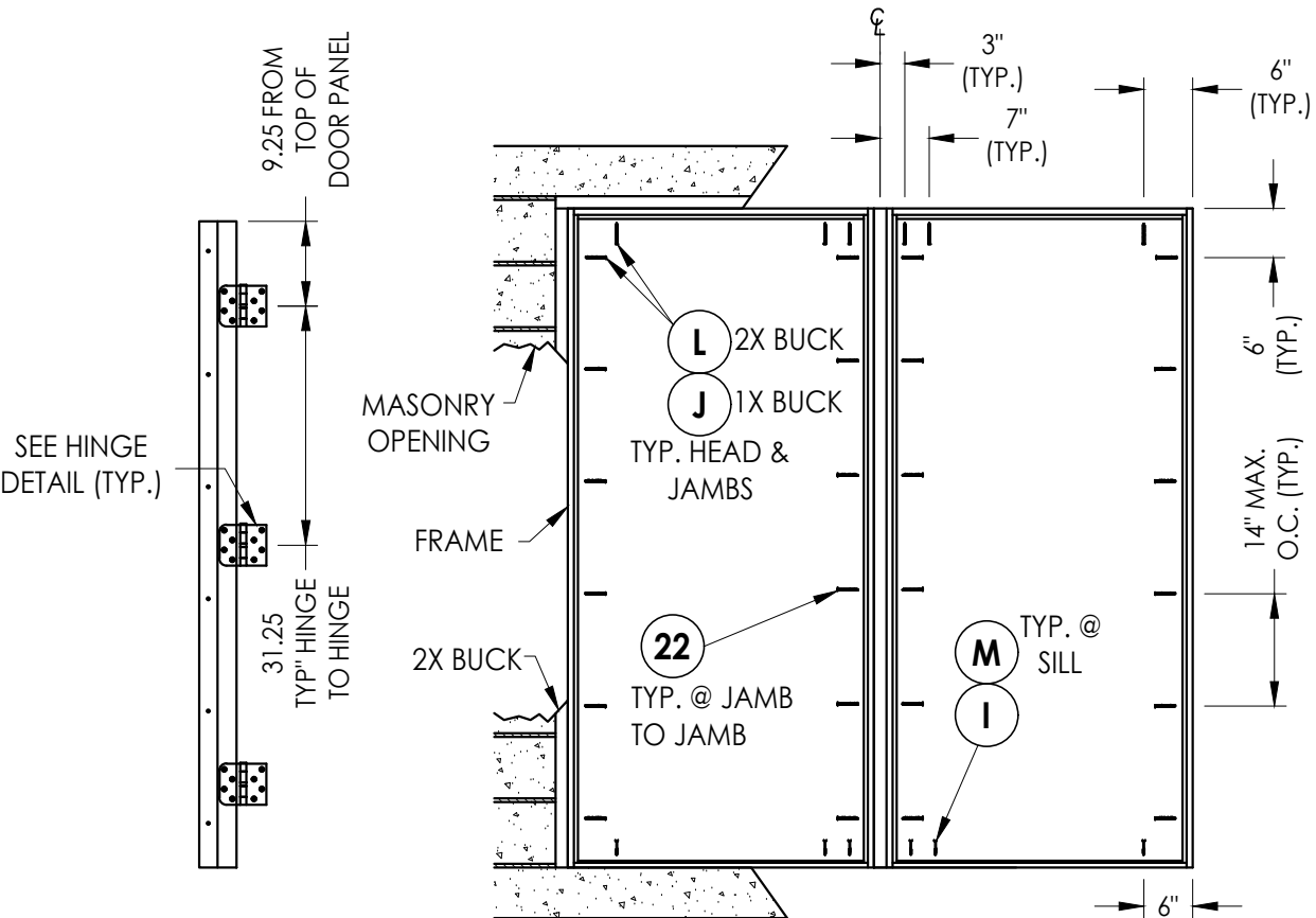
HINGE JAMB
